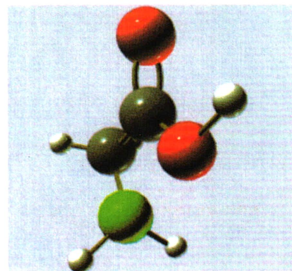
生物大分子的基石——氨基酸
