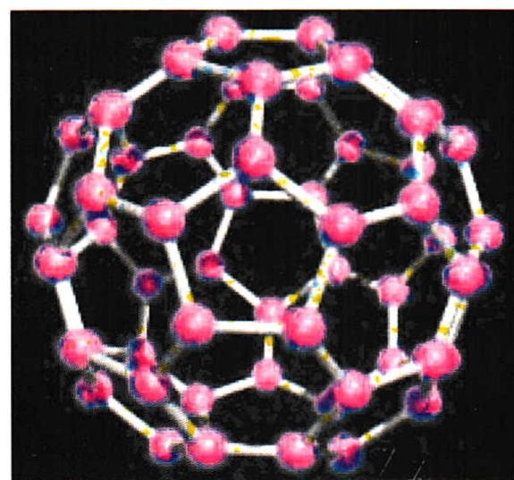
碳60分子结构
