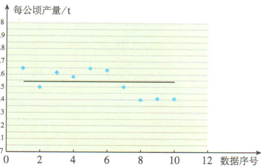
图 20.2-1 甲种甜玉米的产量
